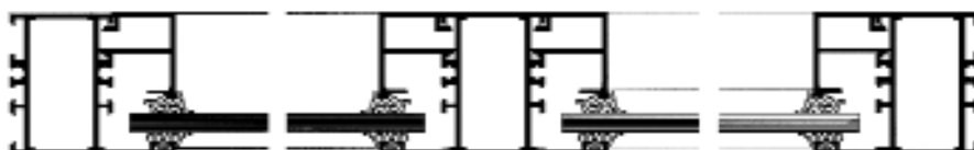
Horizontalschnitt ▲
